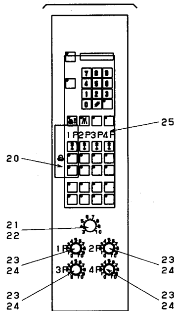
排紙部OP-Sパネル DELIVERY OP-S PANEL NEW TYPE (BW-8L034)
