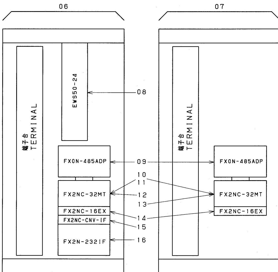
EPS第1制御BOX EPS NO.1 CONTROL BOX
