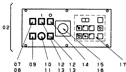
給紙部操作パネル FEEDER SIDE OPERATION PANEL OLD TYPE (~BI-G0034)
